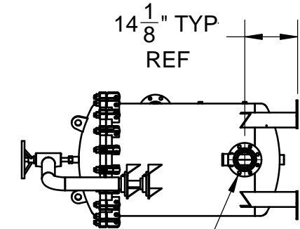
4" ФЛАНЦЕВЫЙ ВЫХОД
